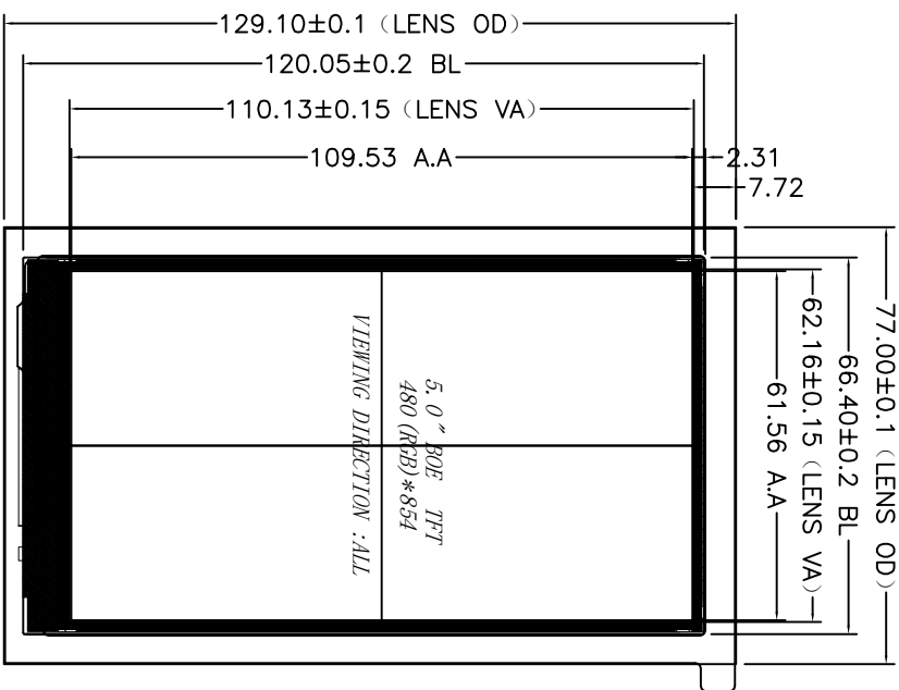
正视图
