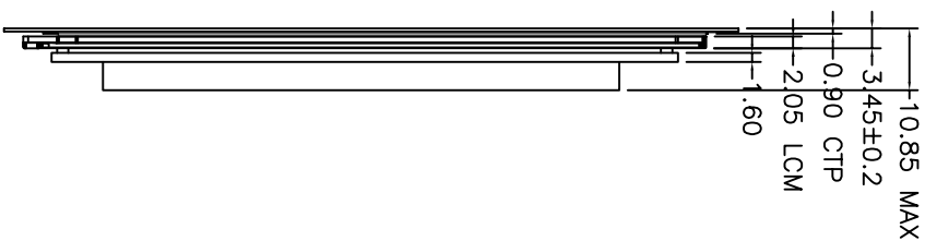
侧视图
