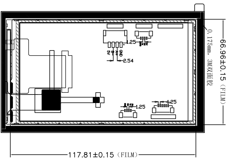
背视图
